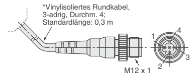
Anschlusskabel mit M12-Steckverbinder (E3ZM-□□□-M1J)
