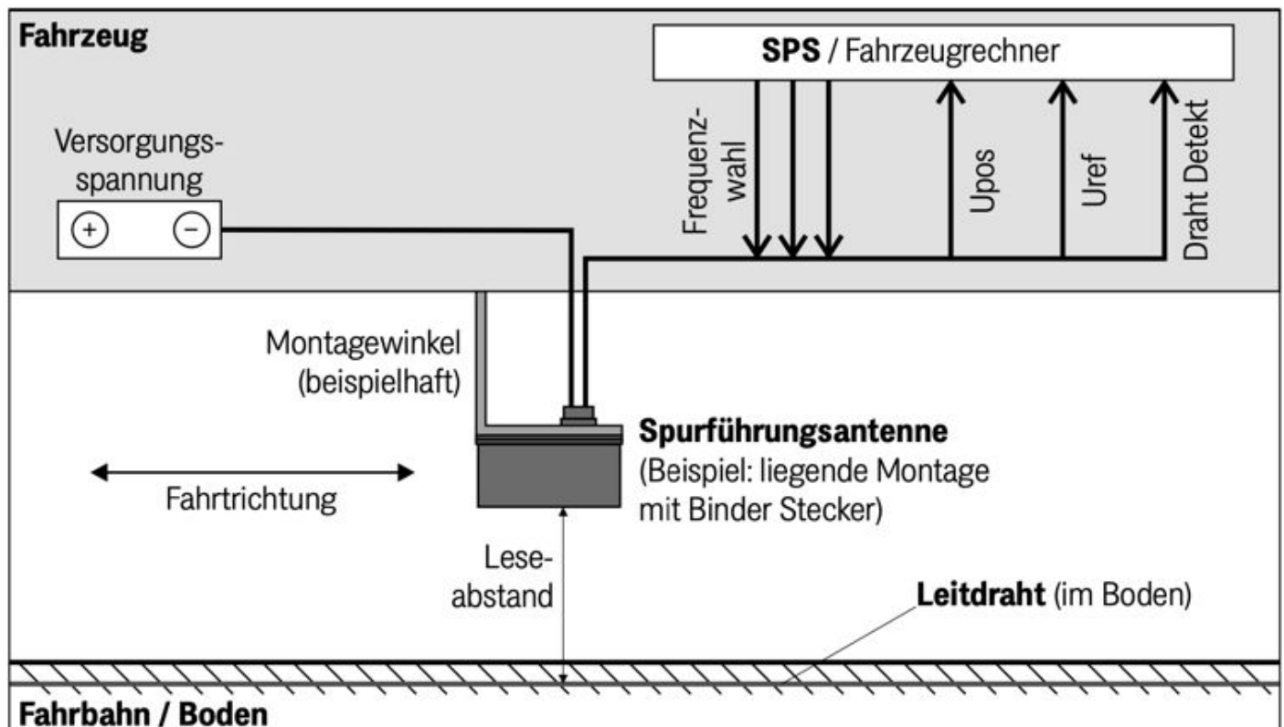
Skizze: Funktionsweise Leitdraht-Spurführung mit Mehrfrequenzsensor HG G-19330-A
