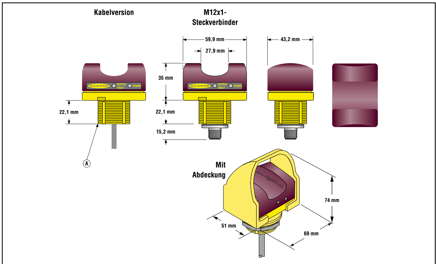
Abb. 7 Abmessungen der STB-Taster
