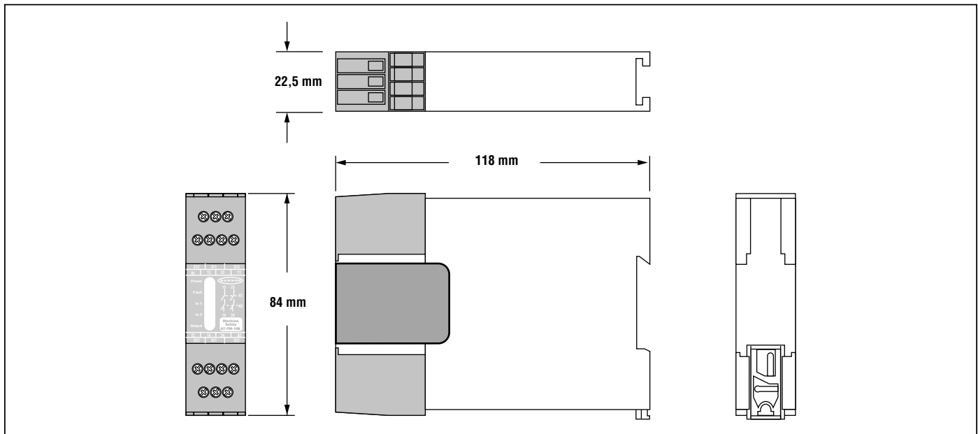
Abb. 6 Abmessungen des DUO-TOUCH SG Sicherheitsmoduls
