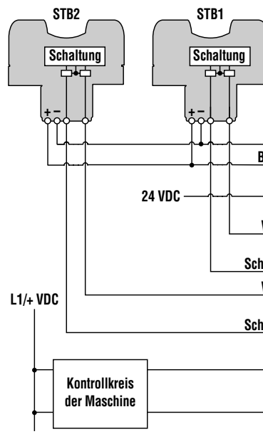
Abb. 5b. Kabelanschluss zwischen dem DUO-TOUCH SG Sicherheitsmodul und zwei STB Tastern mit (stromliefernden) PNP-Ausgängen
