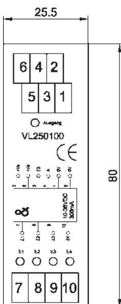
Maßbild
