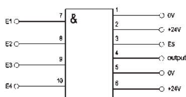
Anschluss UND-Modul
