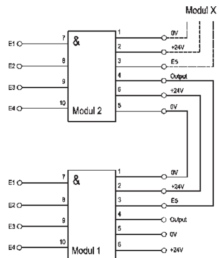
Kaskadierung mehrerer Module
