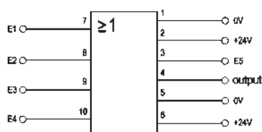
Anschluss ODER-Modul
